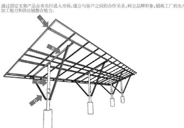
图1 江苏瑞智中和固定式光伏支架结构图
